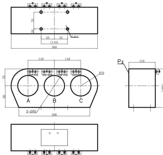
外形图 Outline drawing
